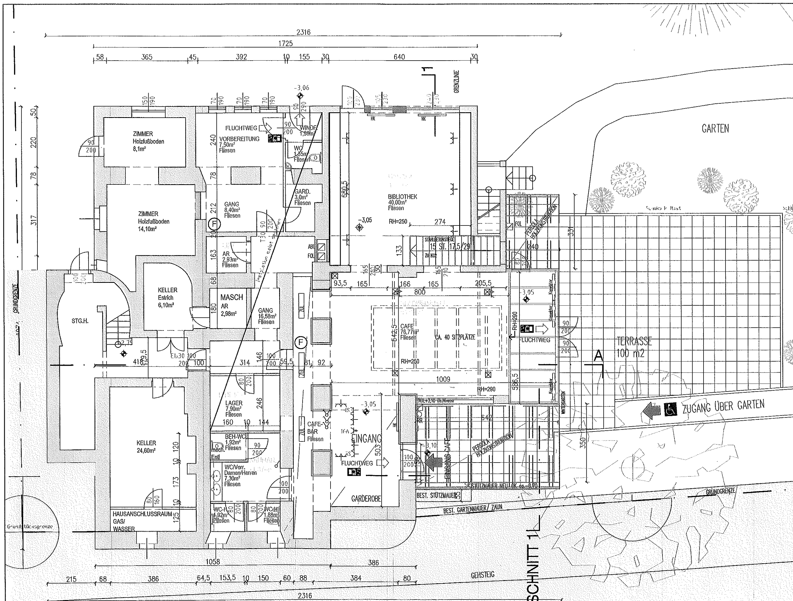
KELLERGEOSCHOSS 1
